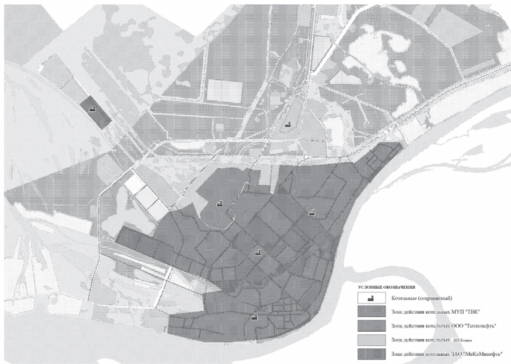
Рисунок 2.4 Схема перспективных зон действия котельных в г. Мегион на расчетный период до 2035 года
