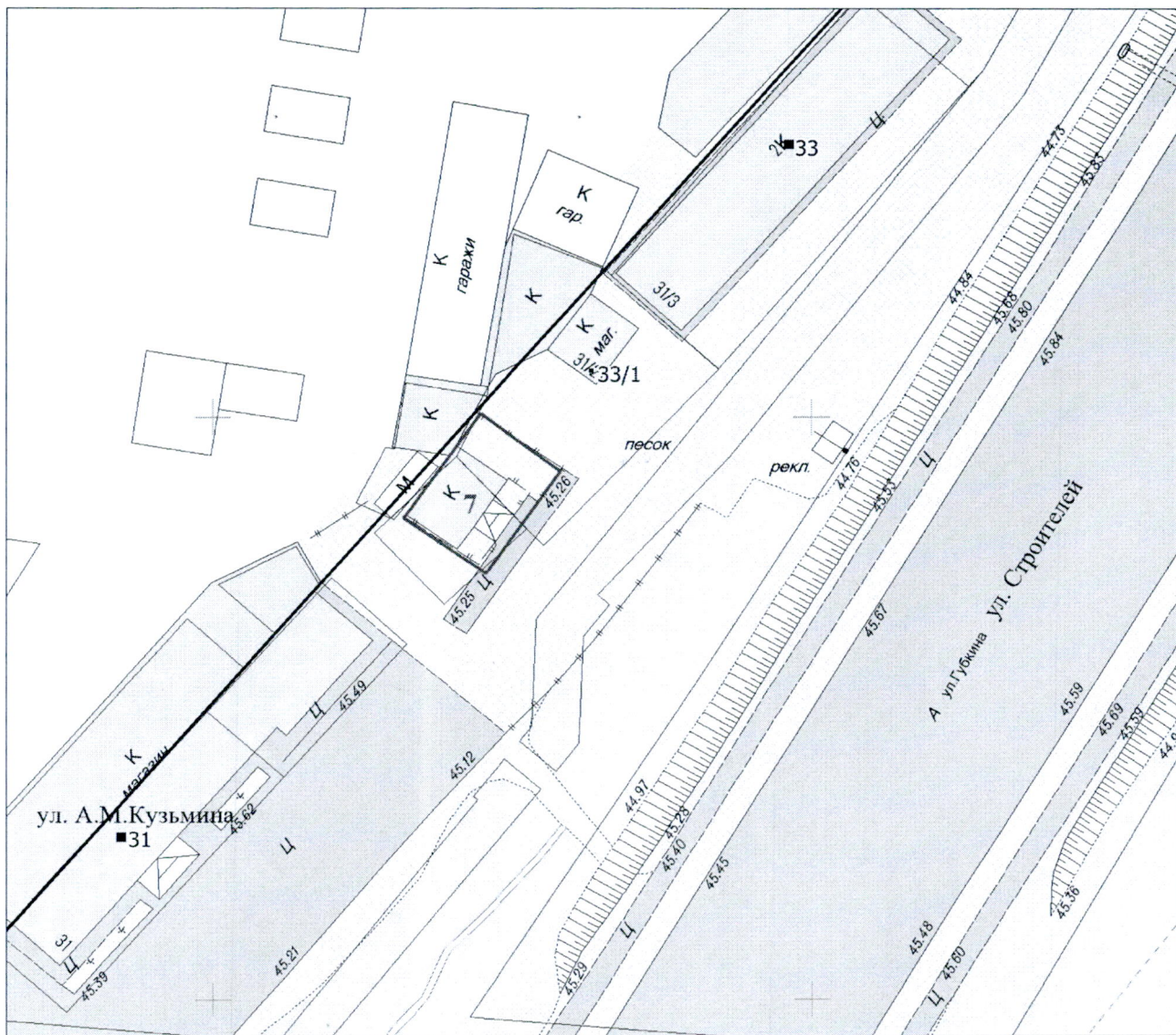
М 1:500
