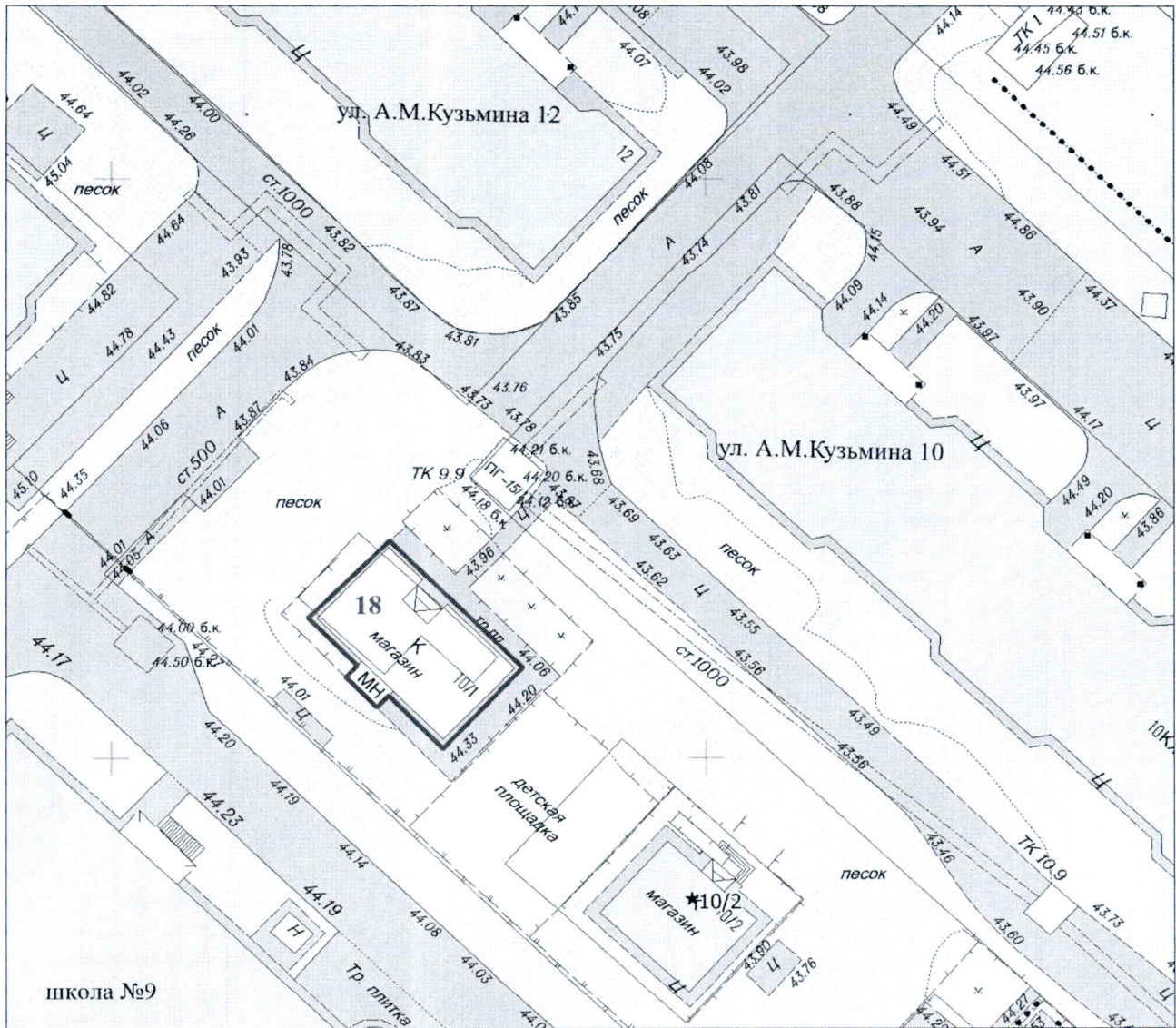
М 1:500
